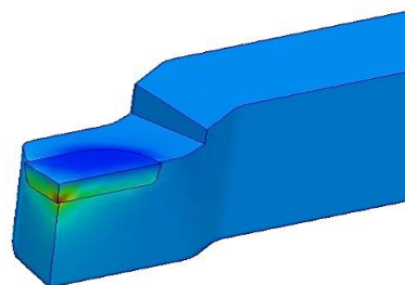
Рисунок 4. Температура пластины резца из твердого сплава ВК8 с охлаждением маслом ПЭ-22 (составлен авторами)
