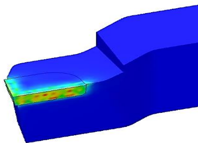
Рисунок 7. Термическое напряжение пластины из быстрорежущей стали Р18 при температуре 217.812^\circ\text{C} составляет 436,522 \text{ МПа}
