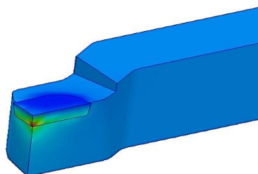
Рисунок 5. Температура пластины из быстрорежущей стали Р18 (составлен авторами)
