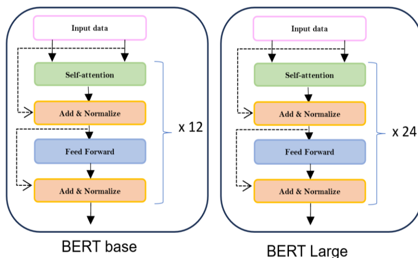
Рисунок 1. Архитектура BERT
